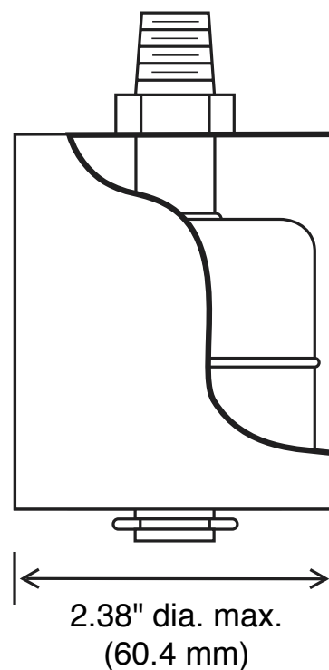
Vue en coupe montrant le fonctionnement de la protection anti ballotement
