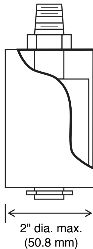
Vue en coupe montrant le fonctionnement de la protection anti ballotement
